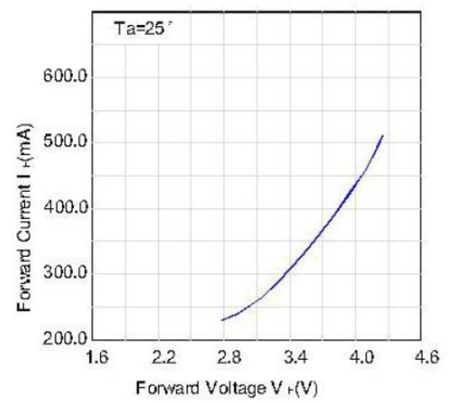
I_f - V_f
